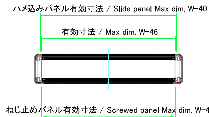
A-A ( 1 : 8 )
